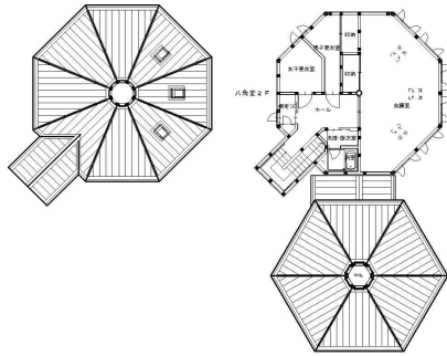
2 階 キープラン S=1/150
